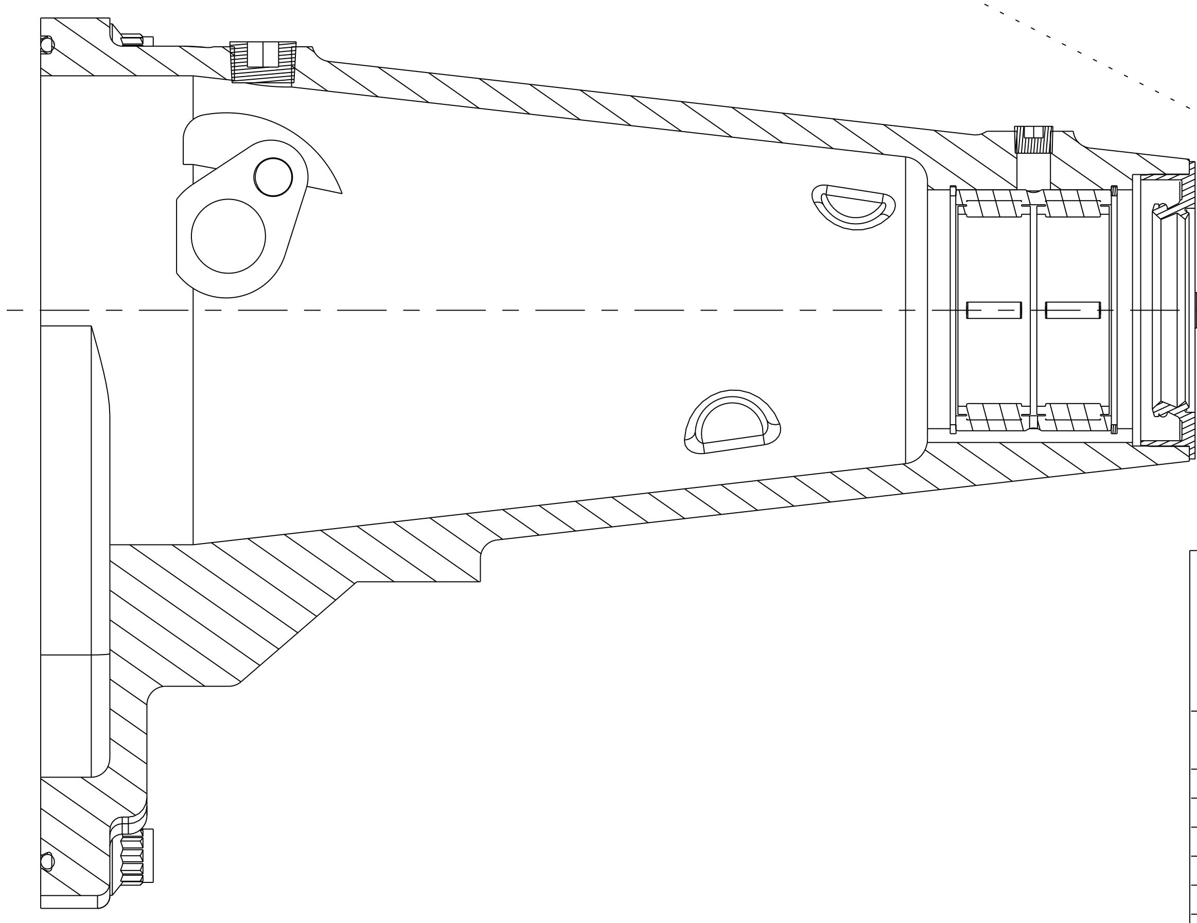
SECTION A-A
